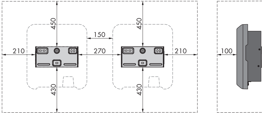
Figure 8 : Distances recommandées (Dimensions en mm)
